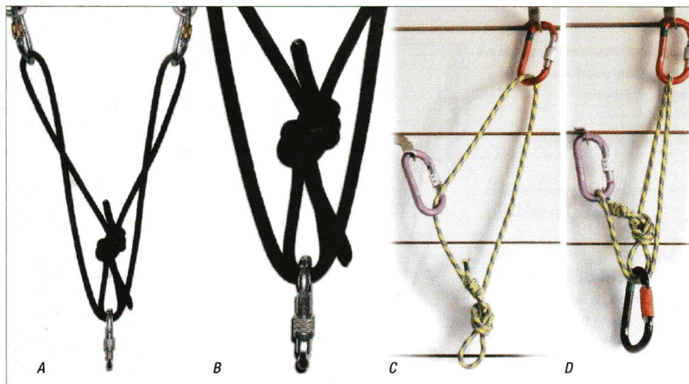
Fig. 4: La sosta ad asola inglobata (A), un particolare del nodo al vertice (B).
