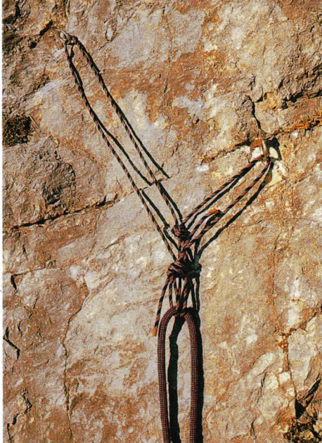
A sinistra: Figura 7 Collegamento a 3 ancoraggi.
