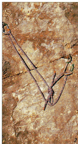
Figura 1 Collegamento classico ancoraggi
